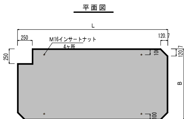
ベースコンクリート寸法図
