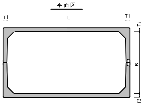
本体寸法図・組立図
