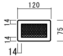
排水用フィルター詳細図
