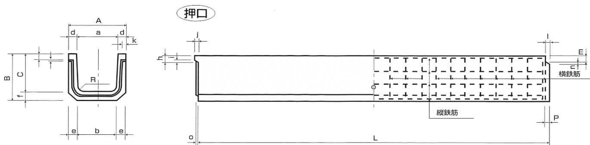
ロングU型形状寸法配筋図
